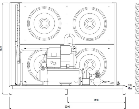
L 2300 x W 1200 x H 1838
